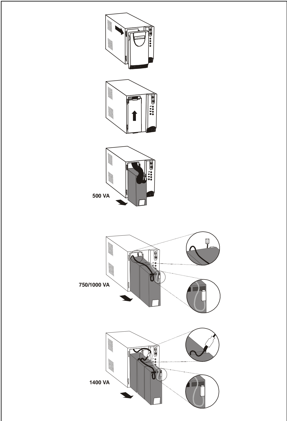
Fig. 9. Remplacement des batteries.
